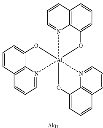
Alq 3
