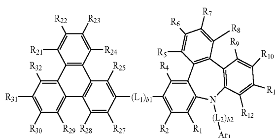
<Formula 1C>
