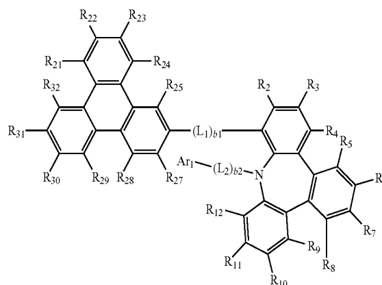
<Formula 1A>
