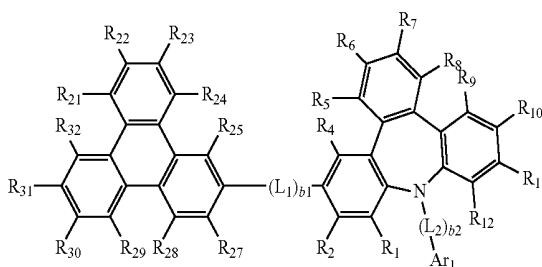
<Formula 1C>
