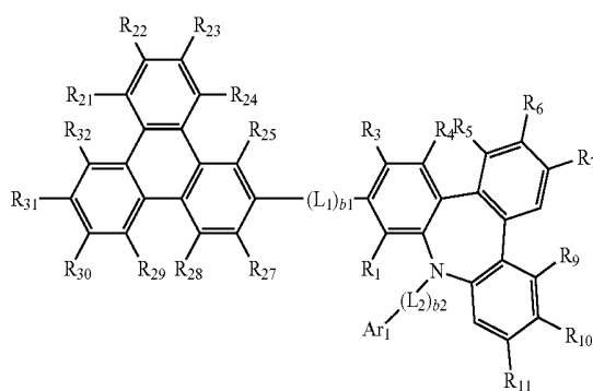
<Formula 1B>
