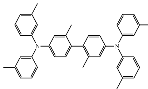
HMTPD
