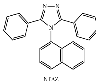
NTAZ
