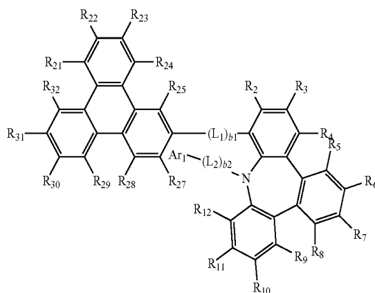
<Formula 1A>
