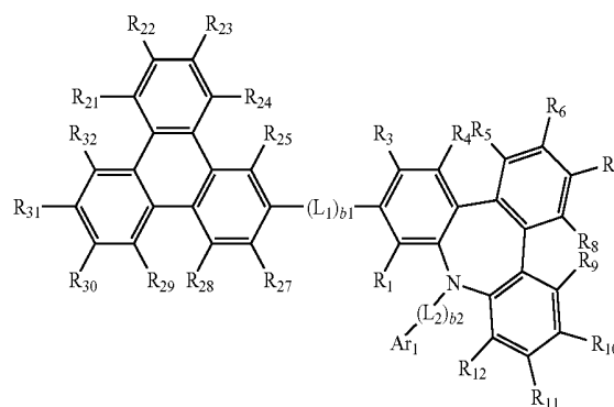
<Formula 1B>
